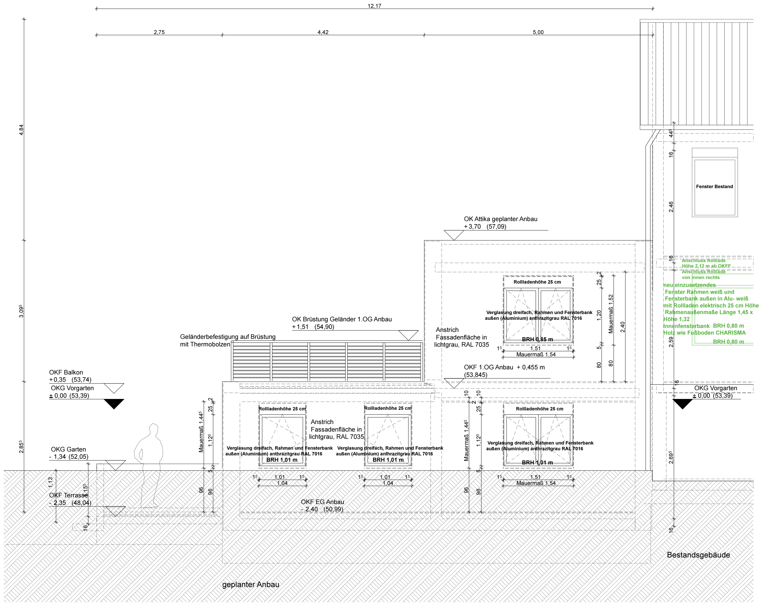
Ansicht Westen
