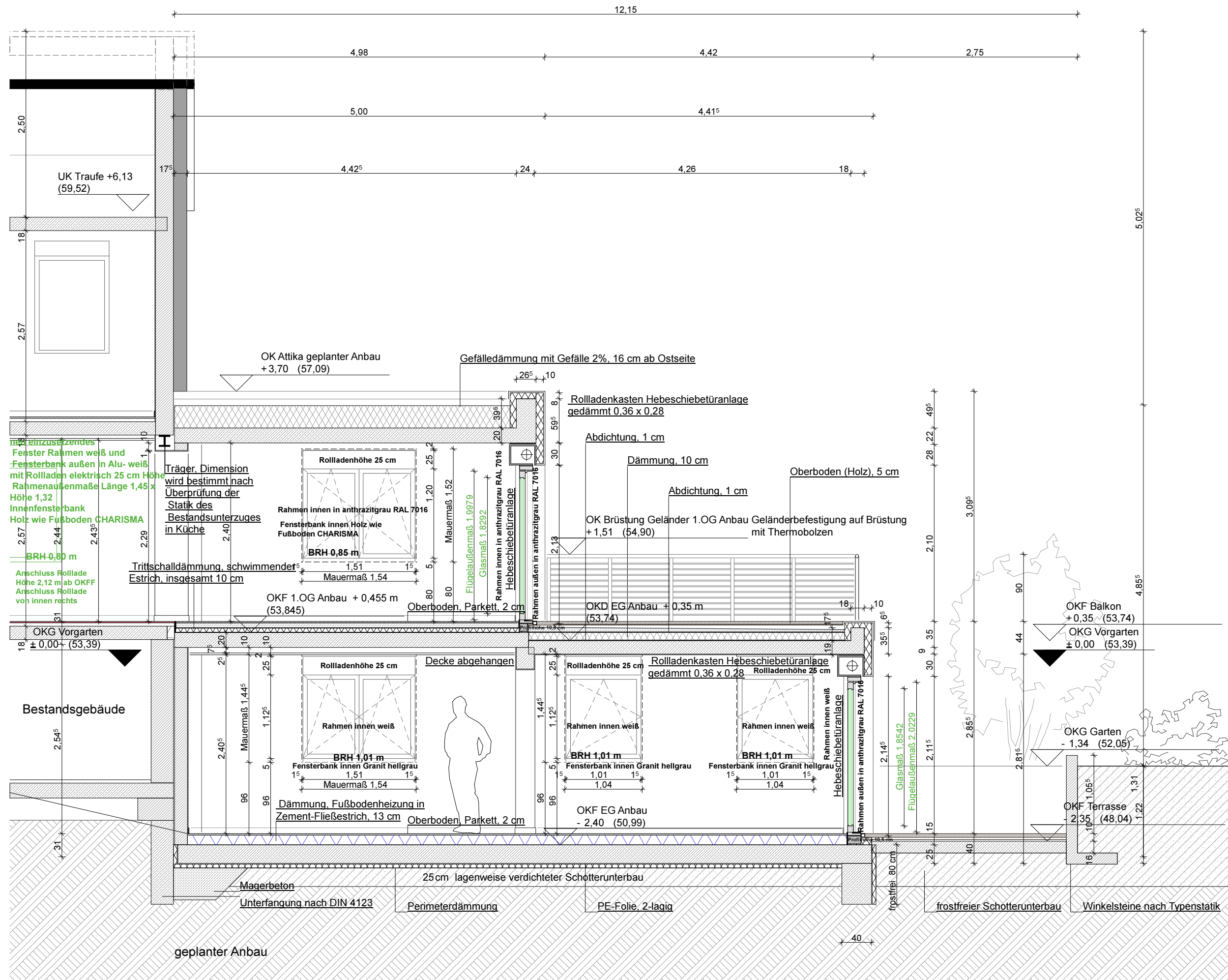
Schnitt A - A
